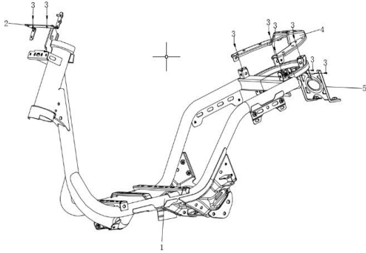
1- CHASIS
