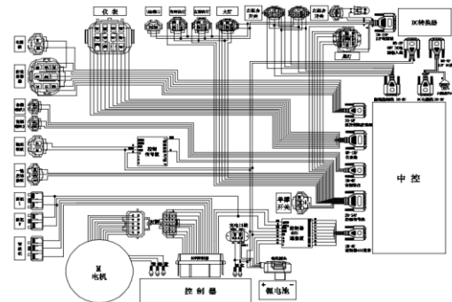
16- CABLEADO ELECTRICO
