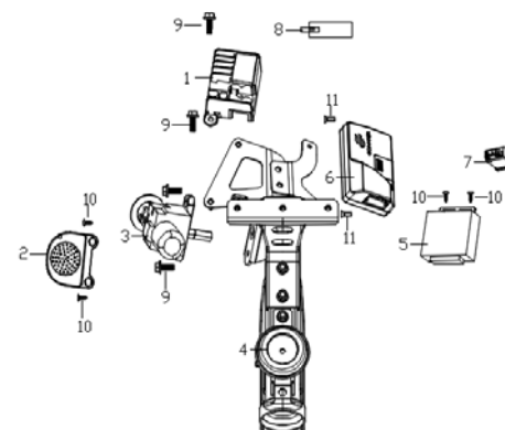
18. Conjunto Cerraduras
