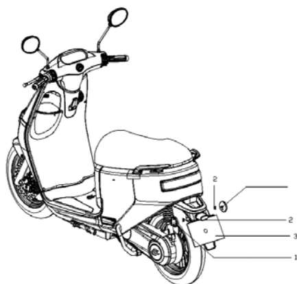
17. Catadioptricos
