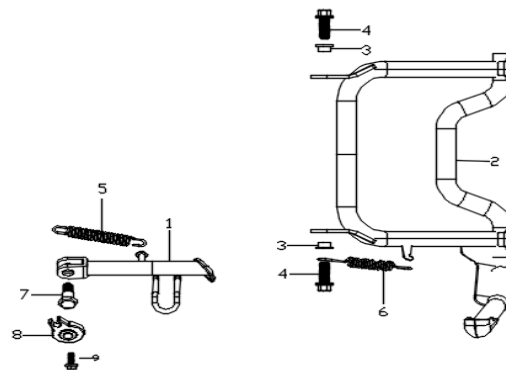
5. Caballetes
