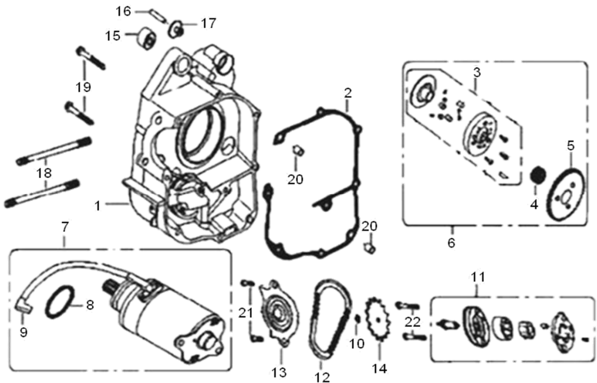
FIG 4 - CARTER DERECHO / BOMBA ACEITE 第5页
