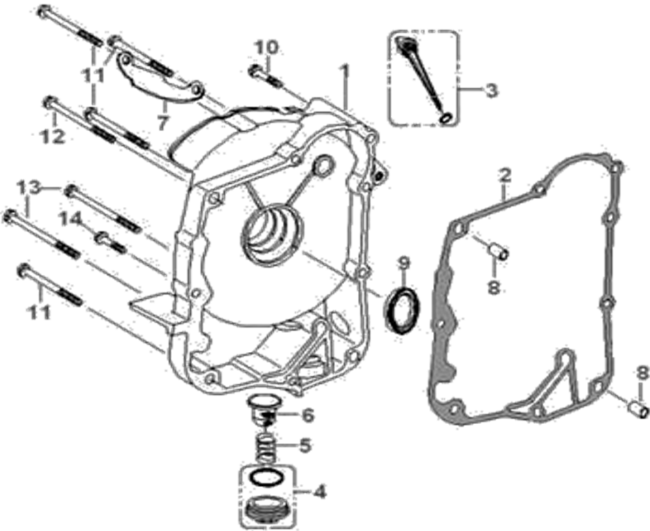
FIG 6 - CARTER DERECHO LADO VOLANTE MAGNETICO ESTATOR 第8页
