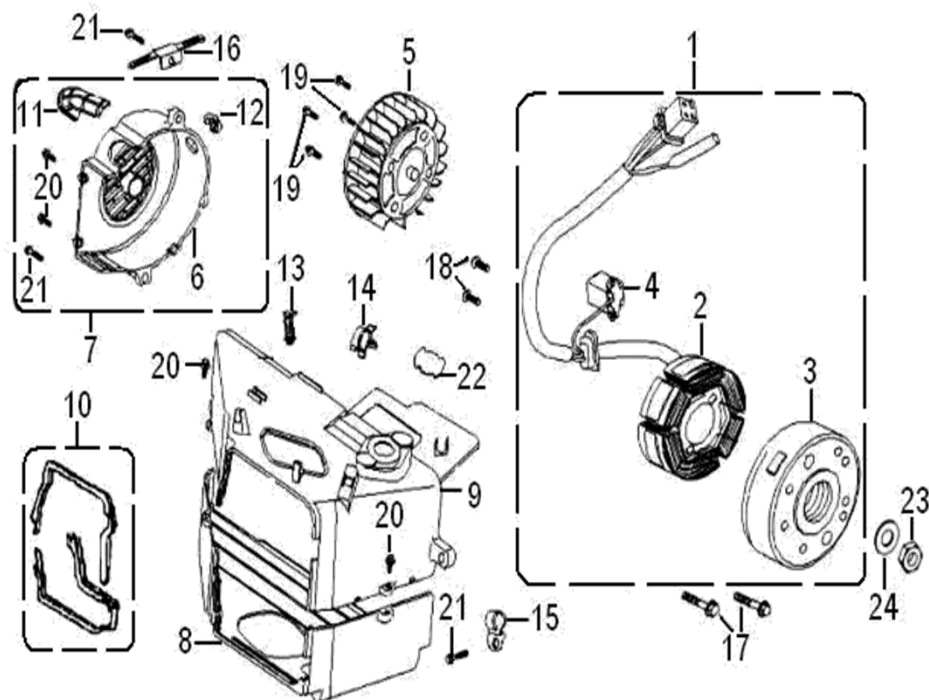
FIG 8 - VENTILADOR &amp; ALTERNATOR
