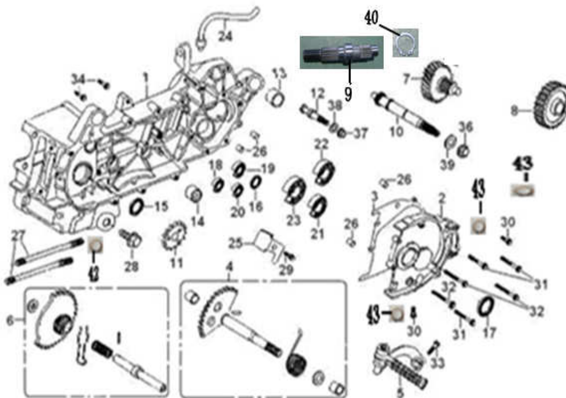
FIG 5 - CARTER IZQUIERDO-PEDAL ARRANQUE-TRANSMISION FINAL
