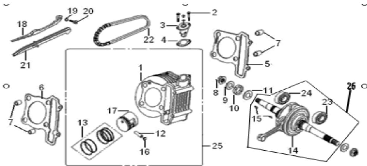
FIG 2 - CILINDER / CILINDRO
