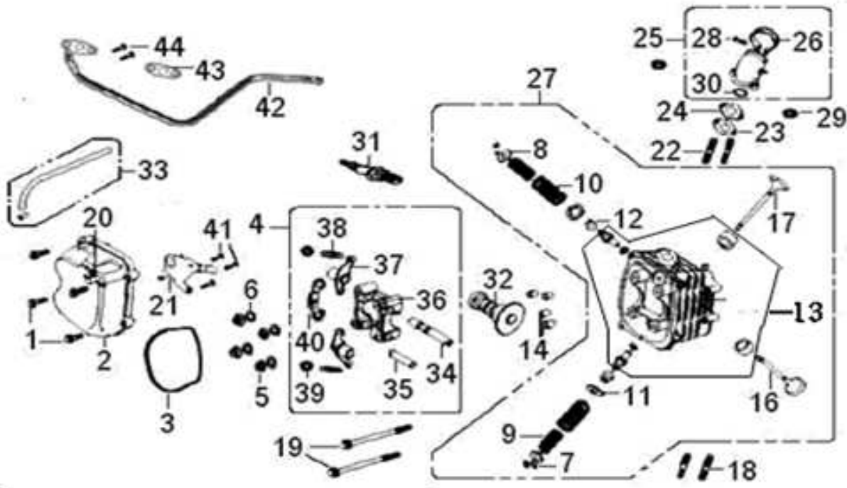
FIG 3 - CYLINDER HEAD / CULATA SISTEMA AIRE SECUNDARIO
