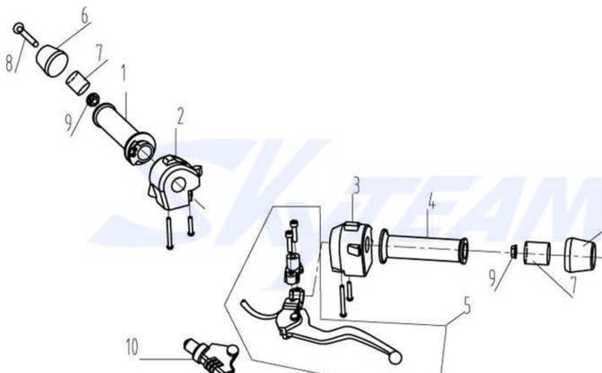
Fig. 1 把手 Handle Bar
