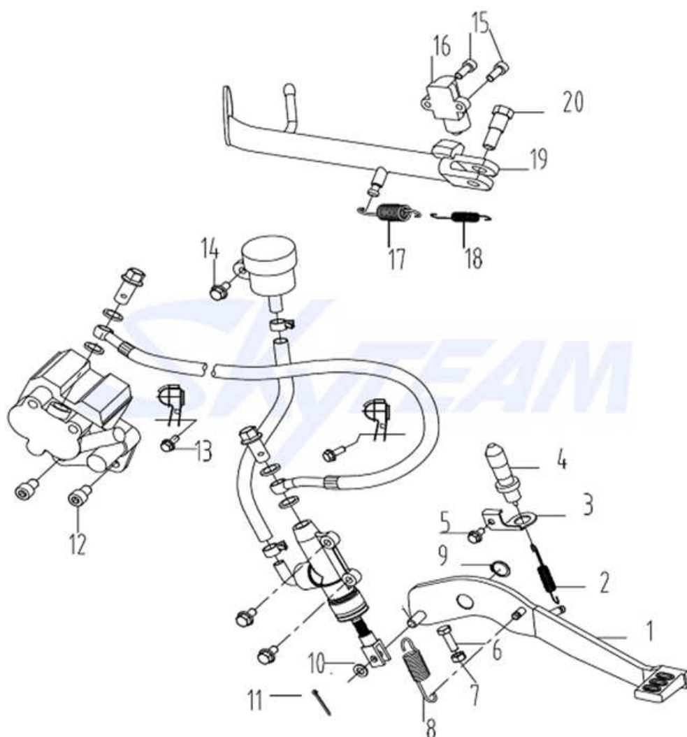
Fig. 10.单撑-后制动 Rear Brake
