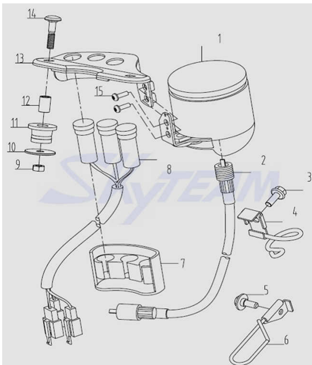
Fig. 3 仪表 Instrument
