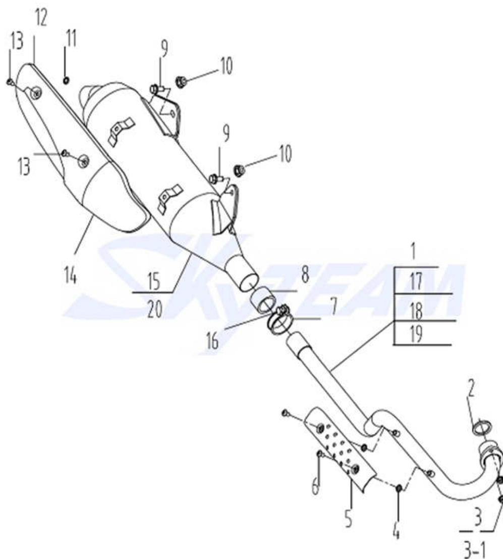
Fig. 16.消音器 Muffler
