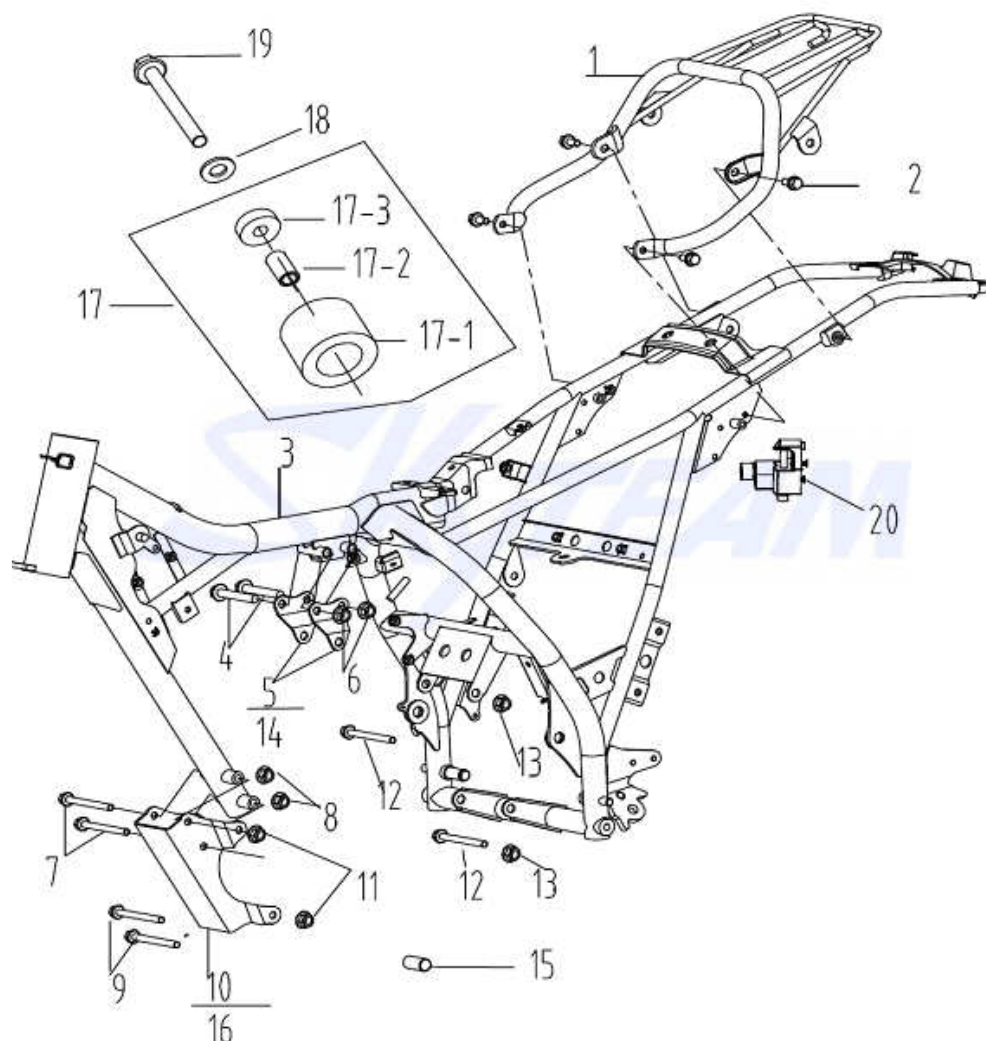
Fig. 11.车架 Frame
