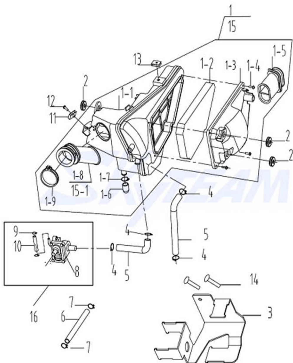
Fig. 14.空滤器 Air Filter
