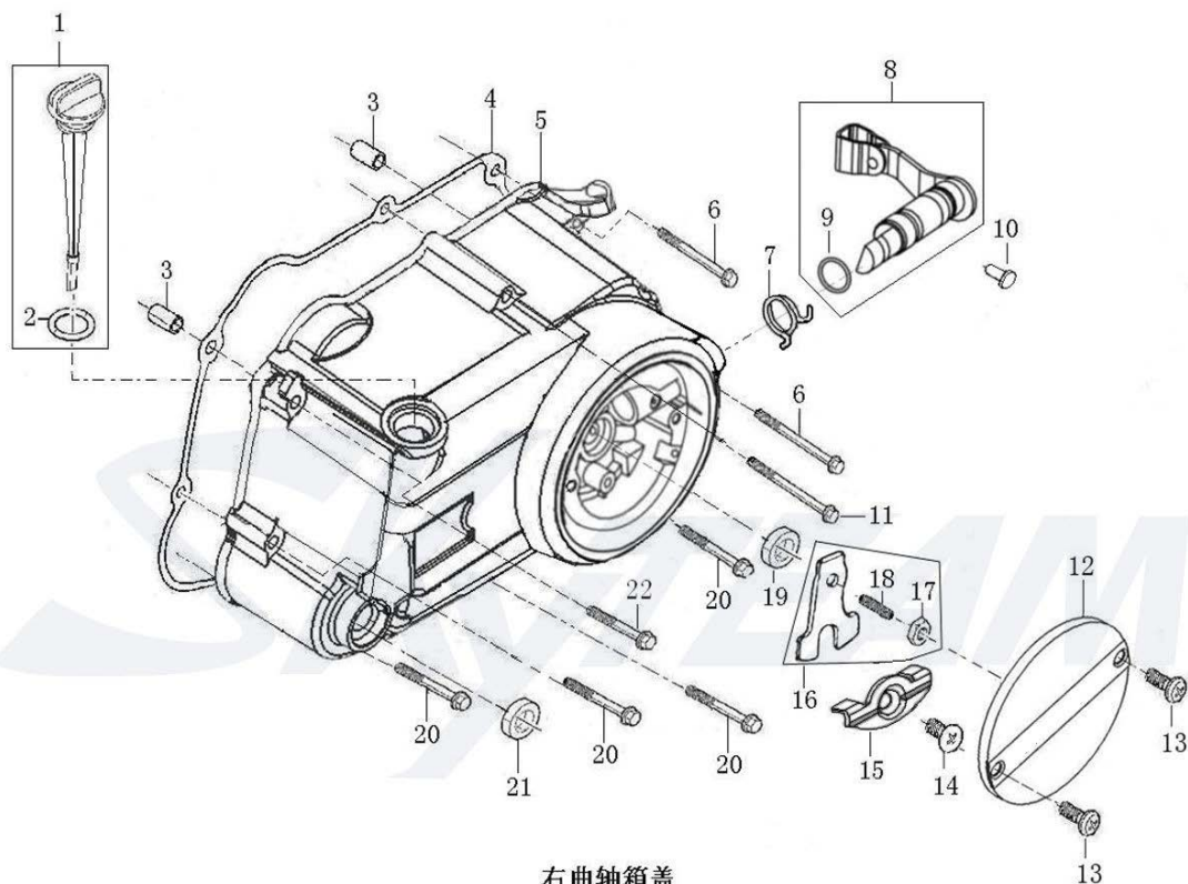
右曲轴箱盖
