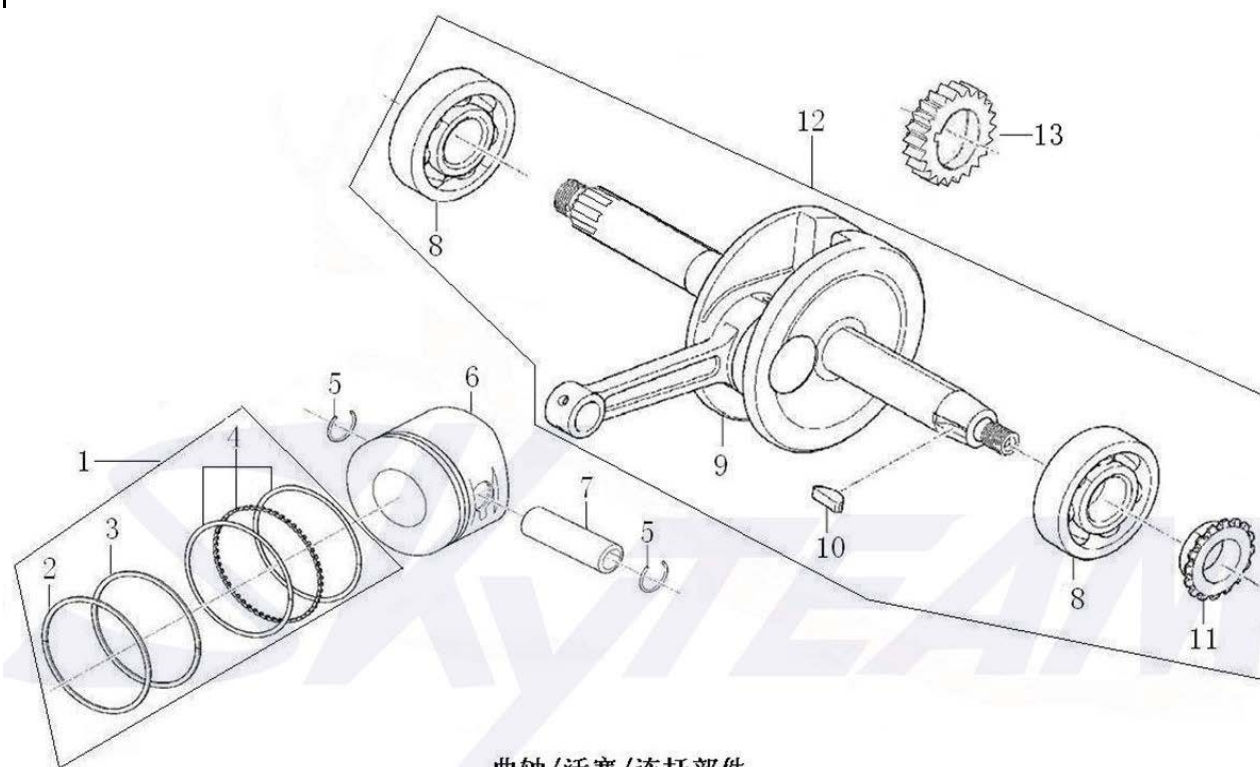
曲轴/活塞/连杆部件
