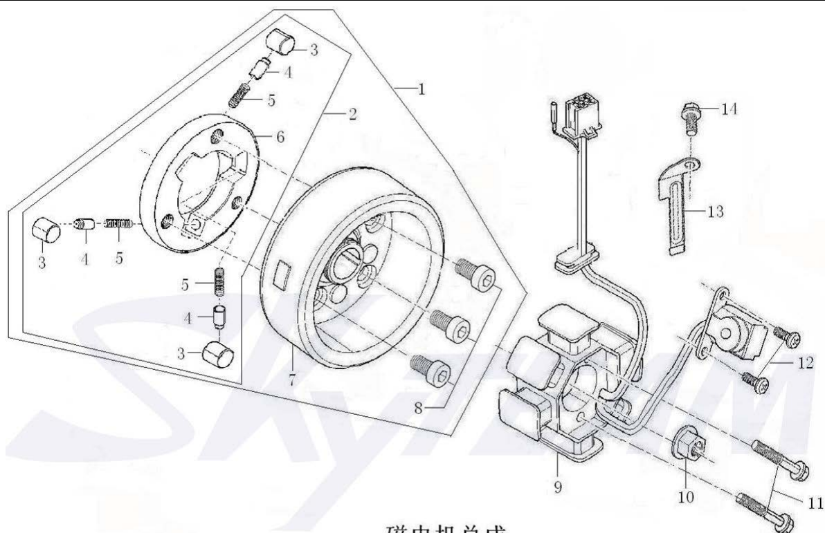
磁中机总成
