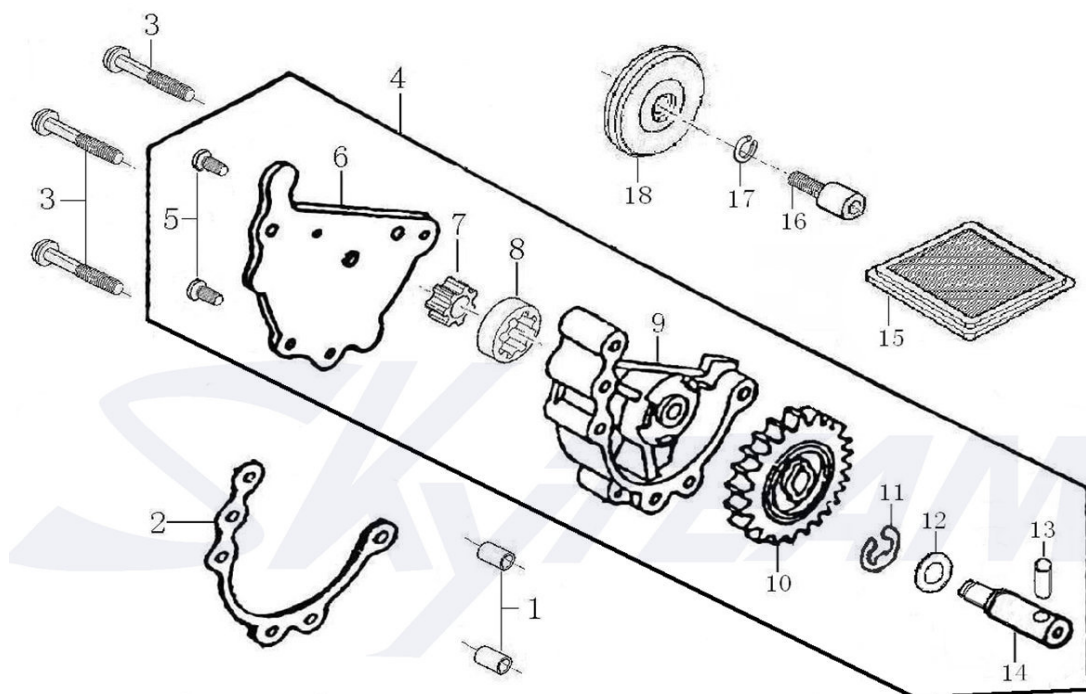
机油泵部件 OIL PUMP
