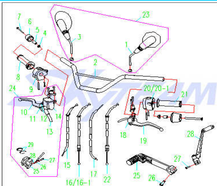
Fig. 6 操纵系统 OPERATION SYSTEM
