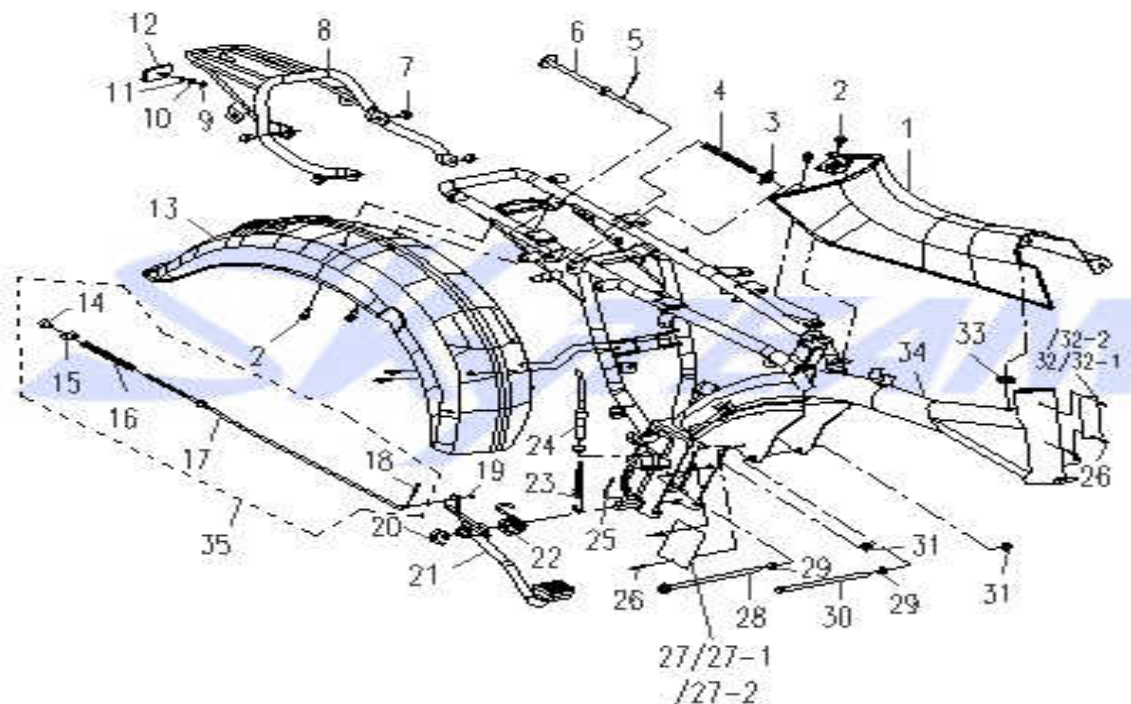
Fig. 8 车架 FRAME-EMBLEM
