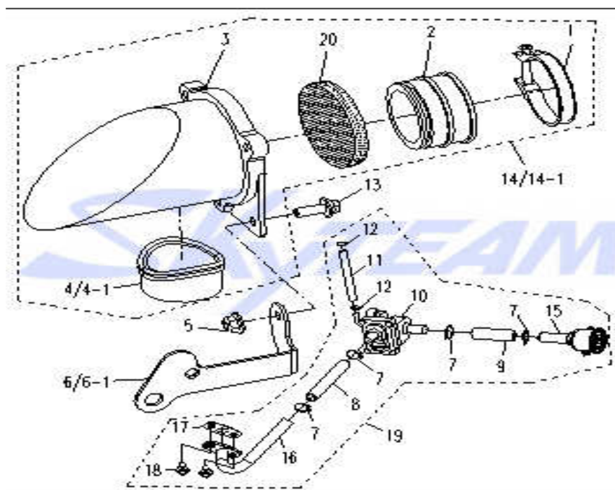
Fig. 4 空滤和二次补气系统 AIR FILTER & SECOND AIR SYSTEM
