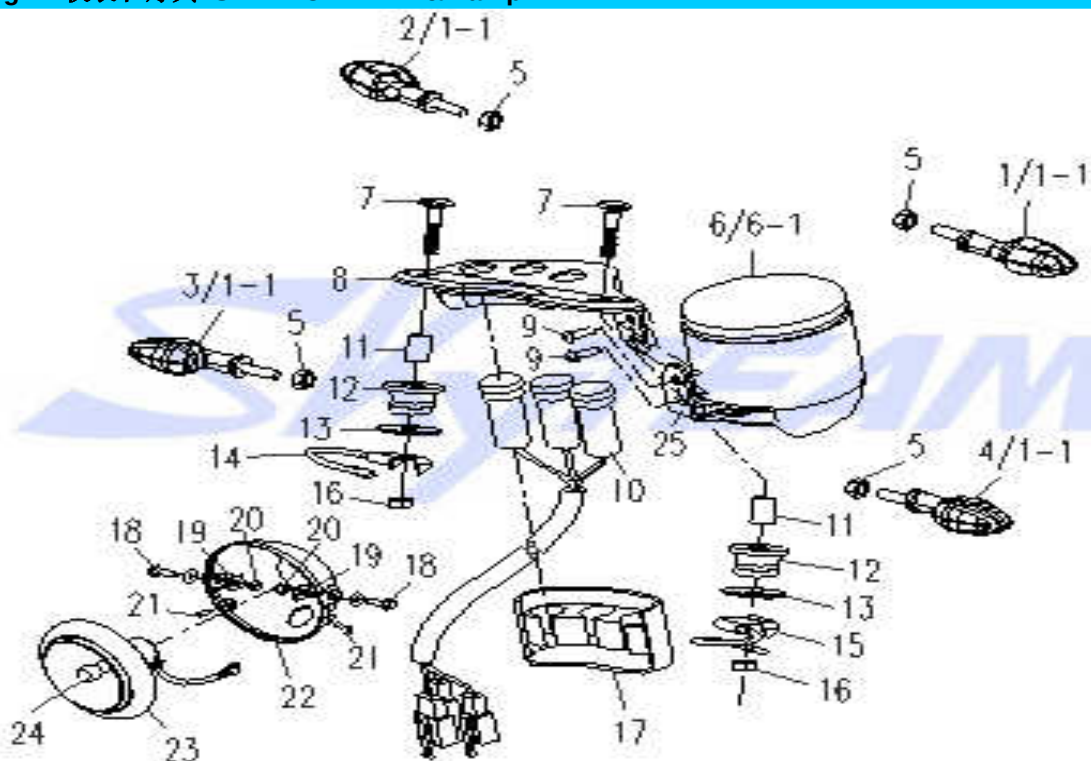
Fig. 2 仪表和灯具 SPEEDOMETER & Lamp
