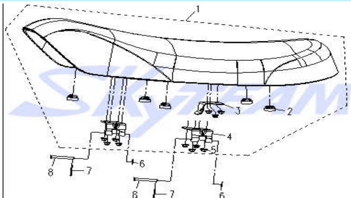
Fig. 10 座垫 SEAT
