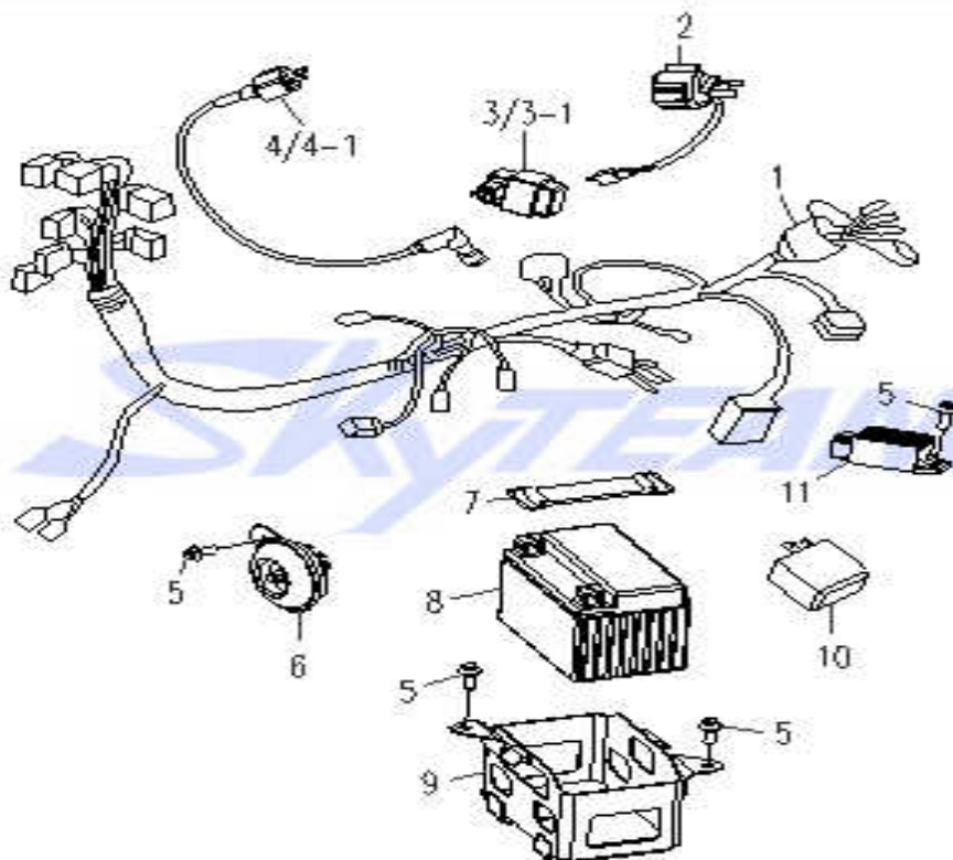
Fig. 1 电器系统 ELECTRICAL COMPONENTS
