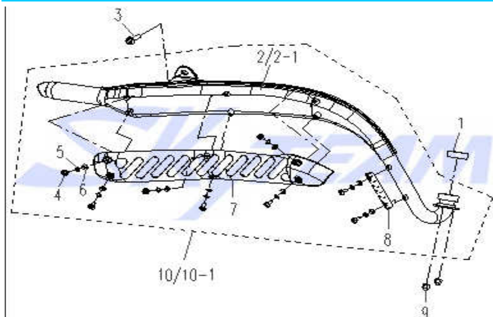
Fig. 5 消音器 MUFFLER ASSY
