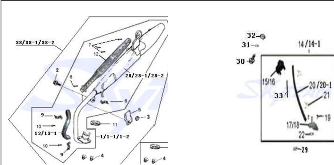
FIG.2 MUFFLER
