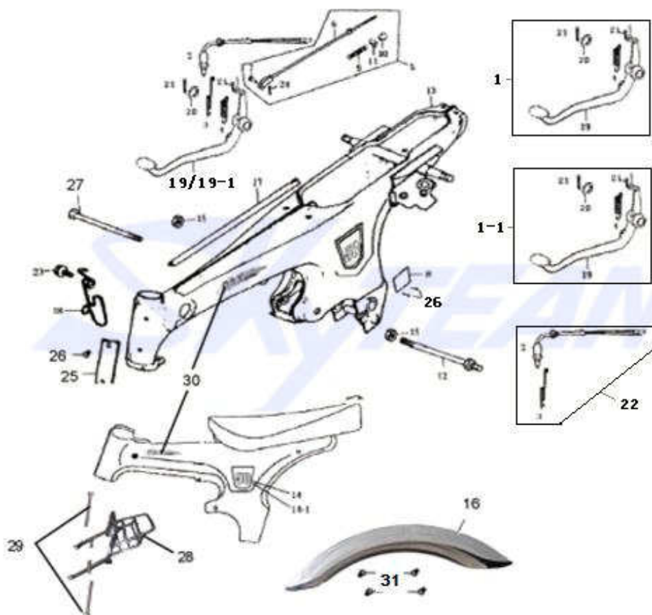
FIG. 15 FRAME-EMBLEM
